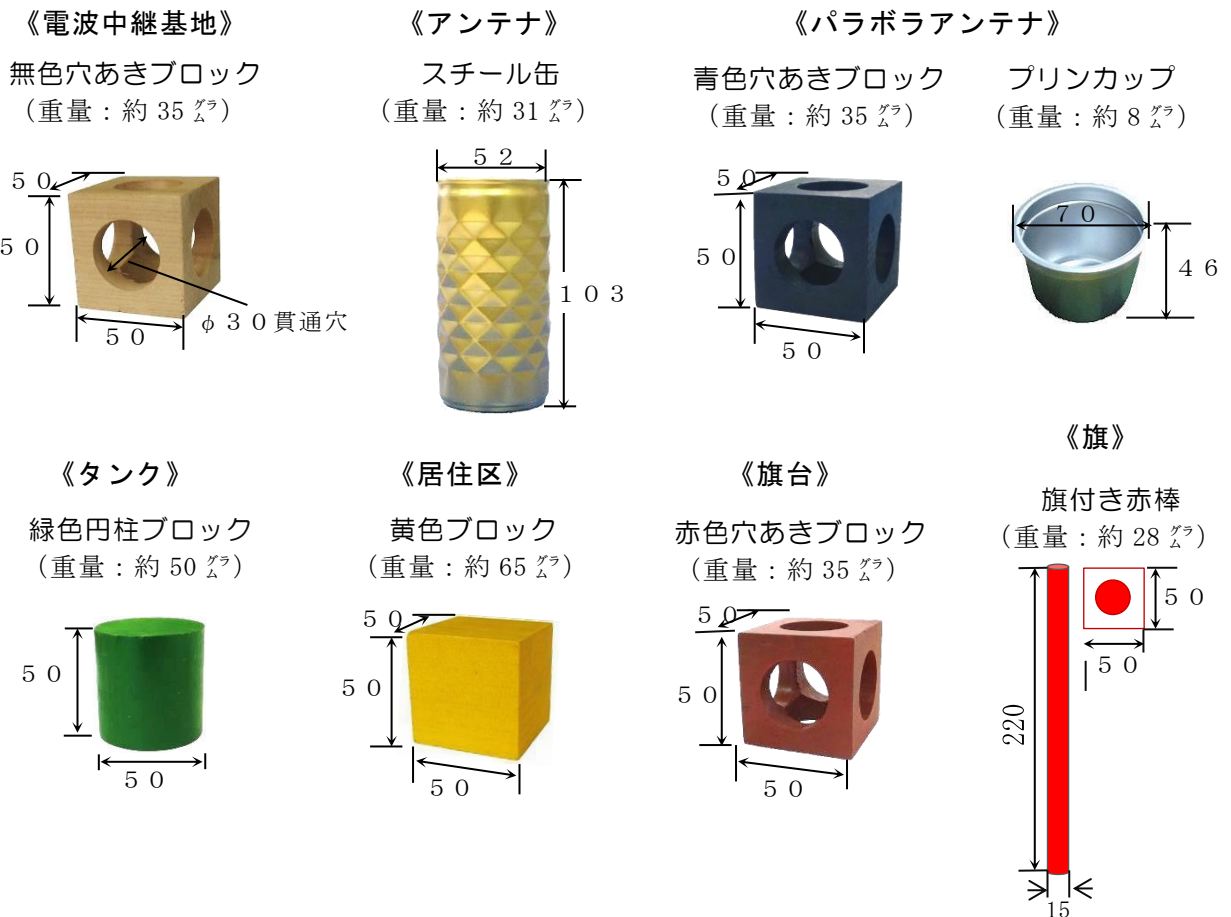
図3. アイテムの外形と寸法・重量
