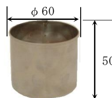
資源コンテナ内土台 (重量：約 22 ｇ)
