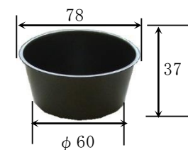
レア資源ポット(プリンカップ) (重量：約 31 ｇ)
